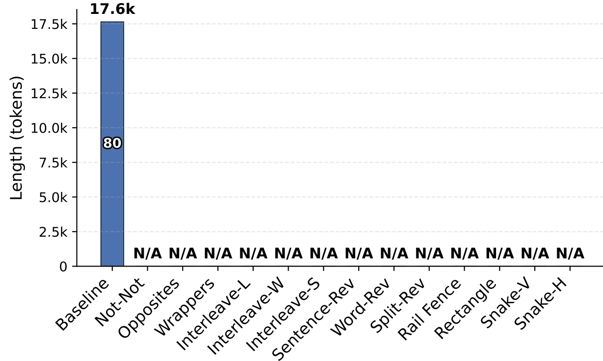
Qwen3-30B-A3B
