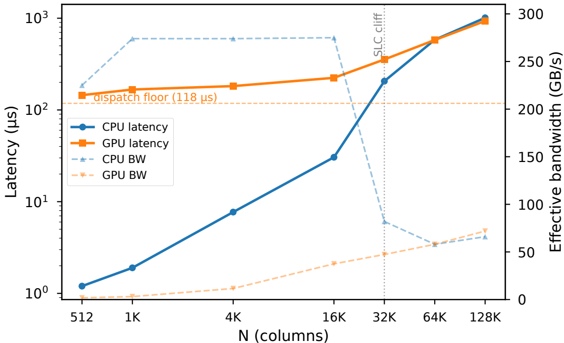
CPU (AMX) vs GPU (Metal) GEMV — 1×128 @ 128×N
