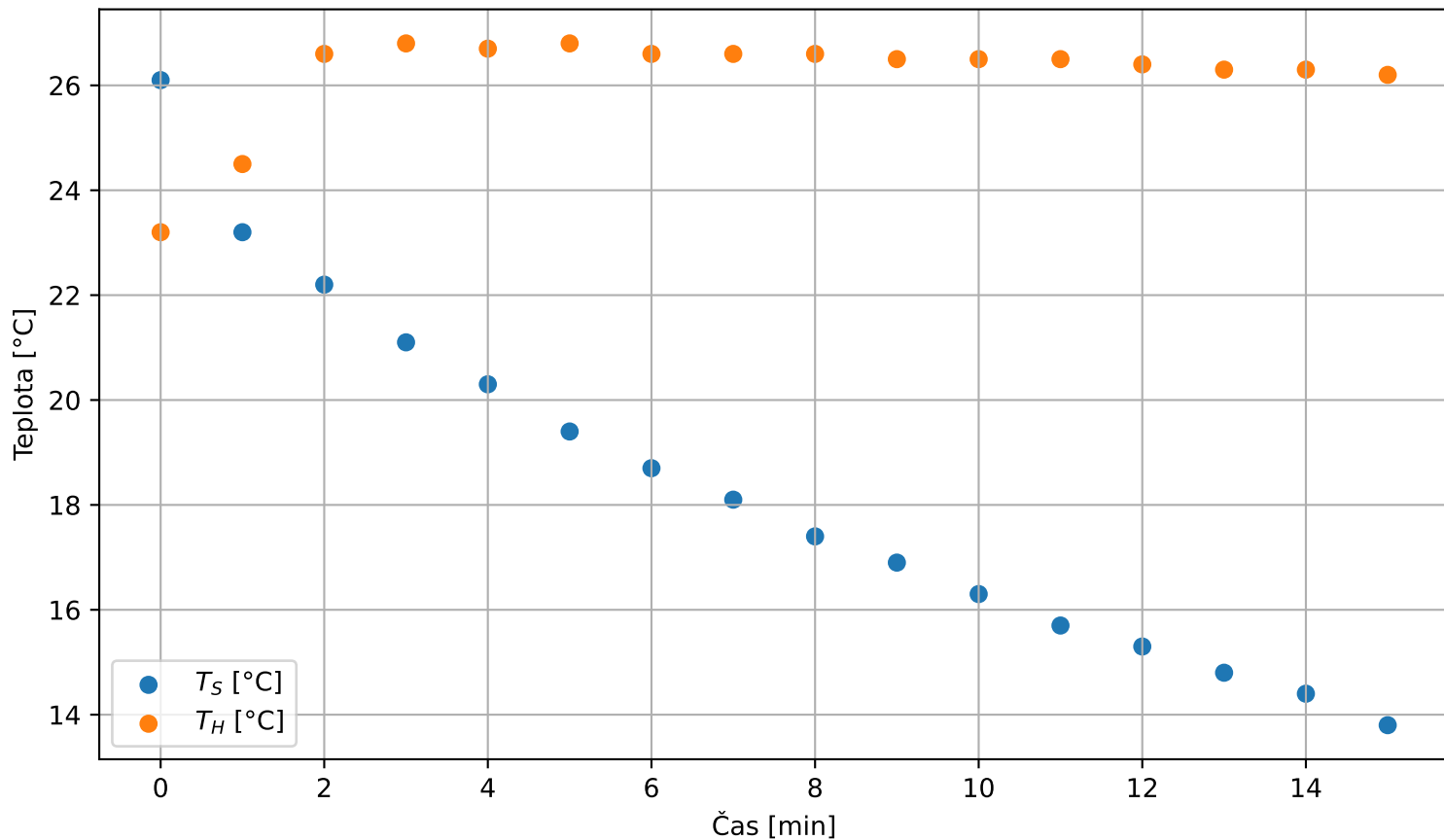
Teploty T_S a T_H v čase (režim TEC)
