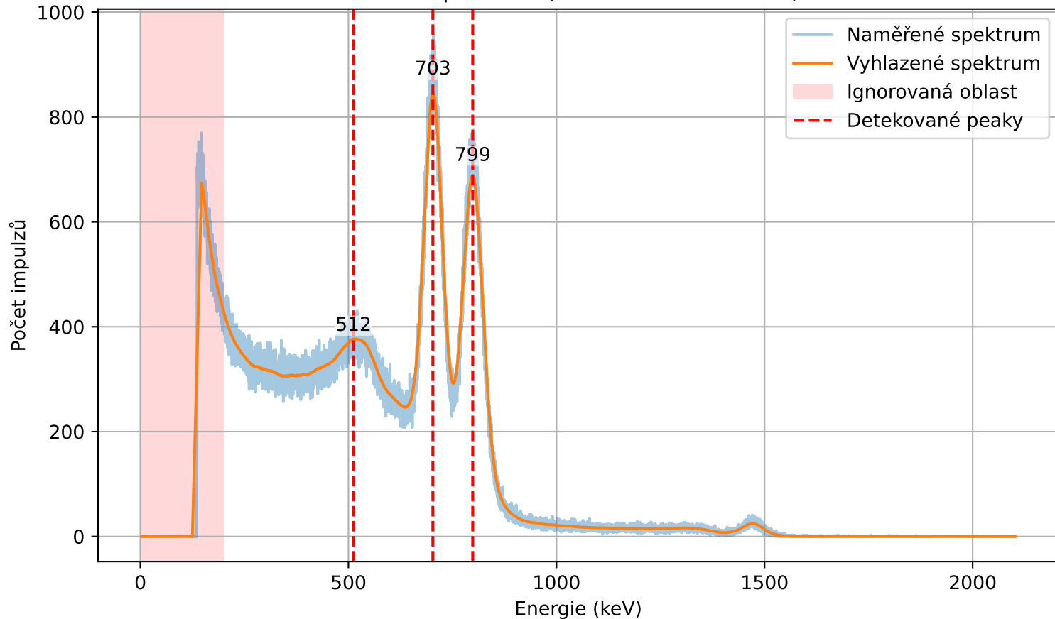
Gama spektrum (Cobalt 60 - měření 1)
