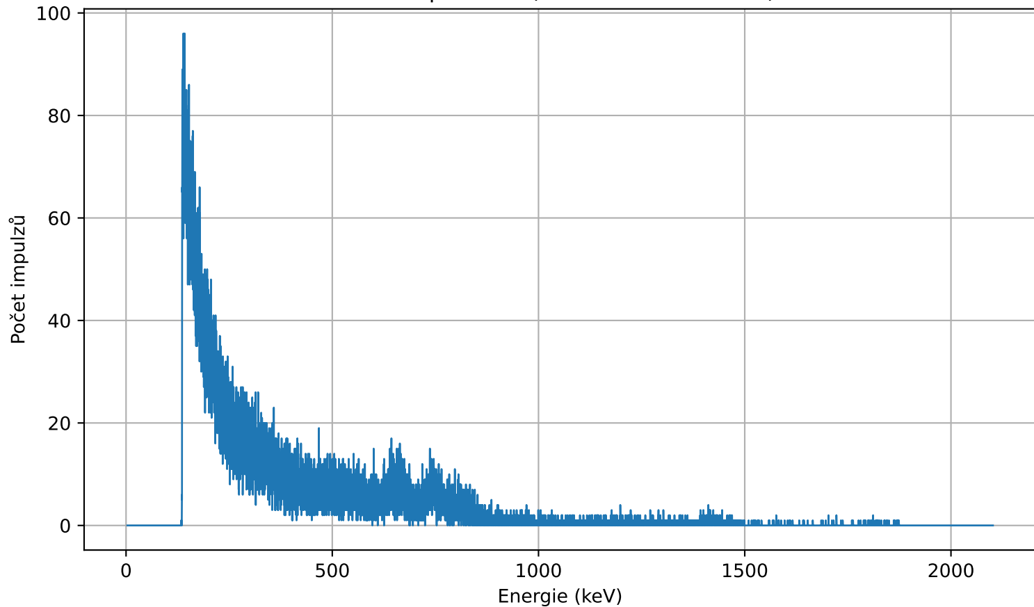
Gama spektrum (Cobalt 60 - měření 2)
