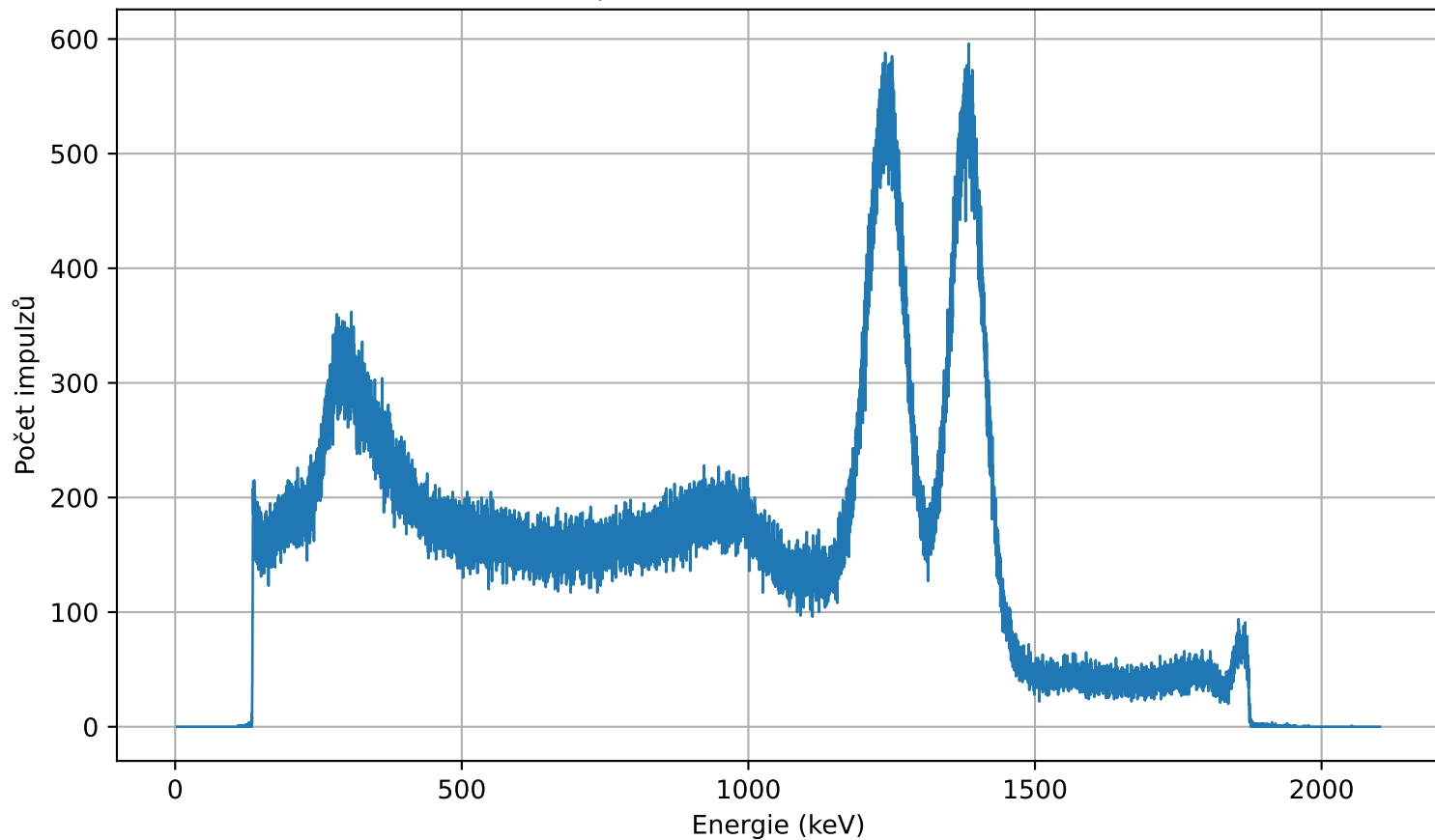
Gama spektrum (Cobalt 60 - měření 3)
