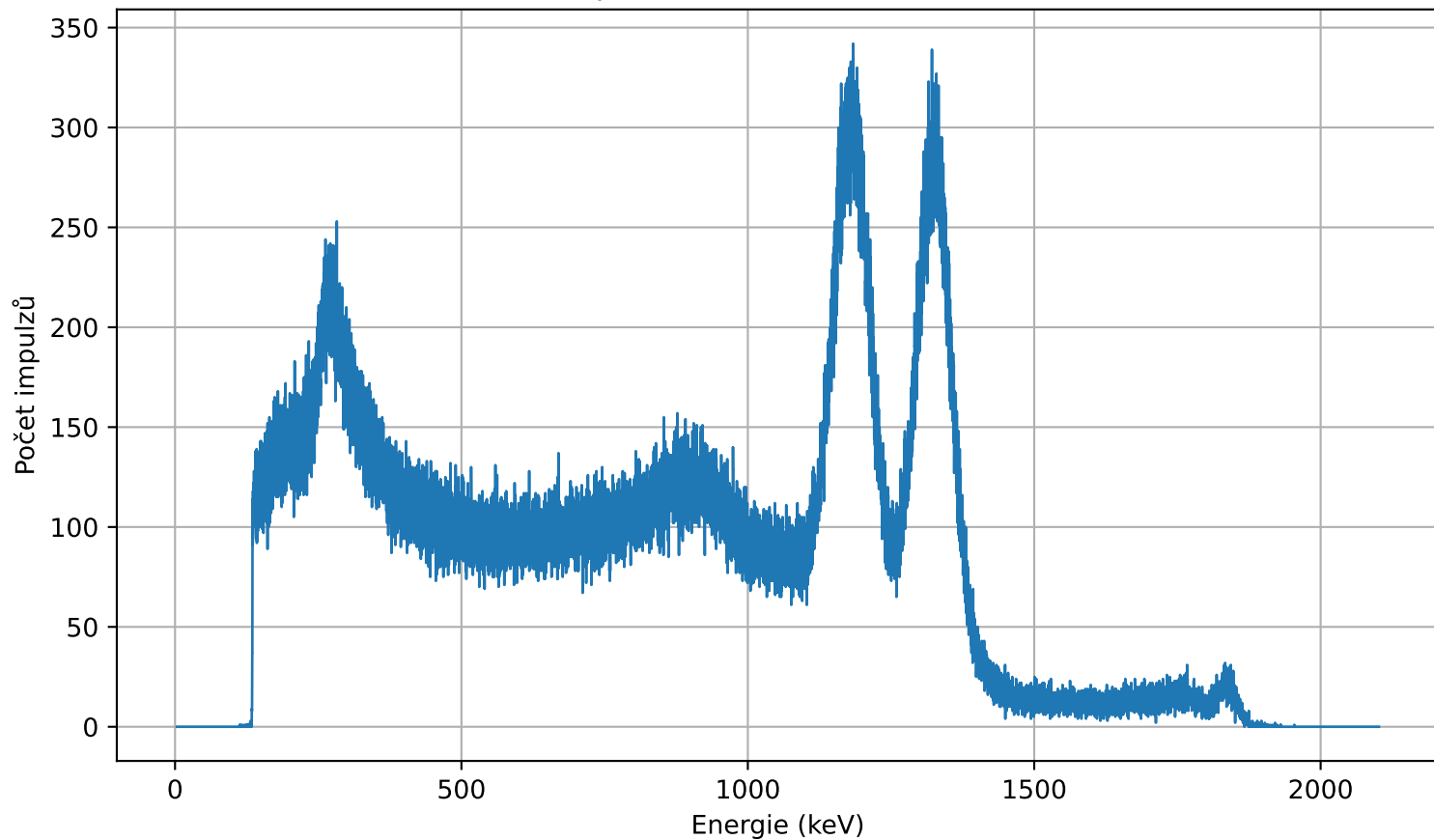
Gama spektrum (Cobalt 60 - měření 4)
