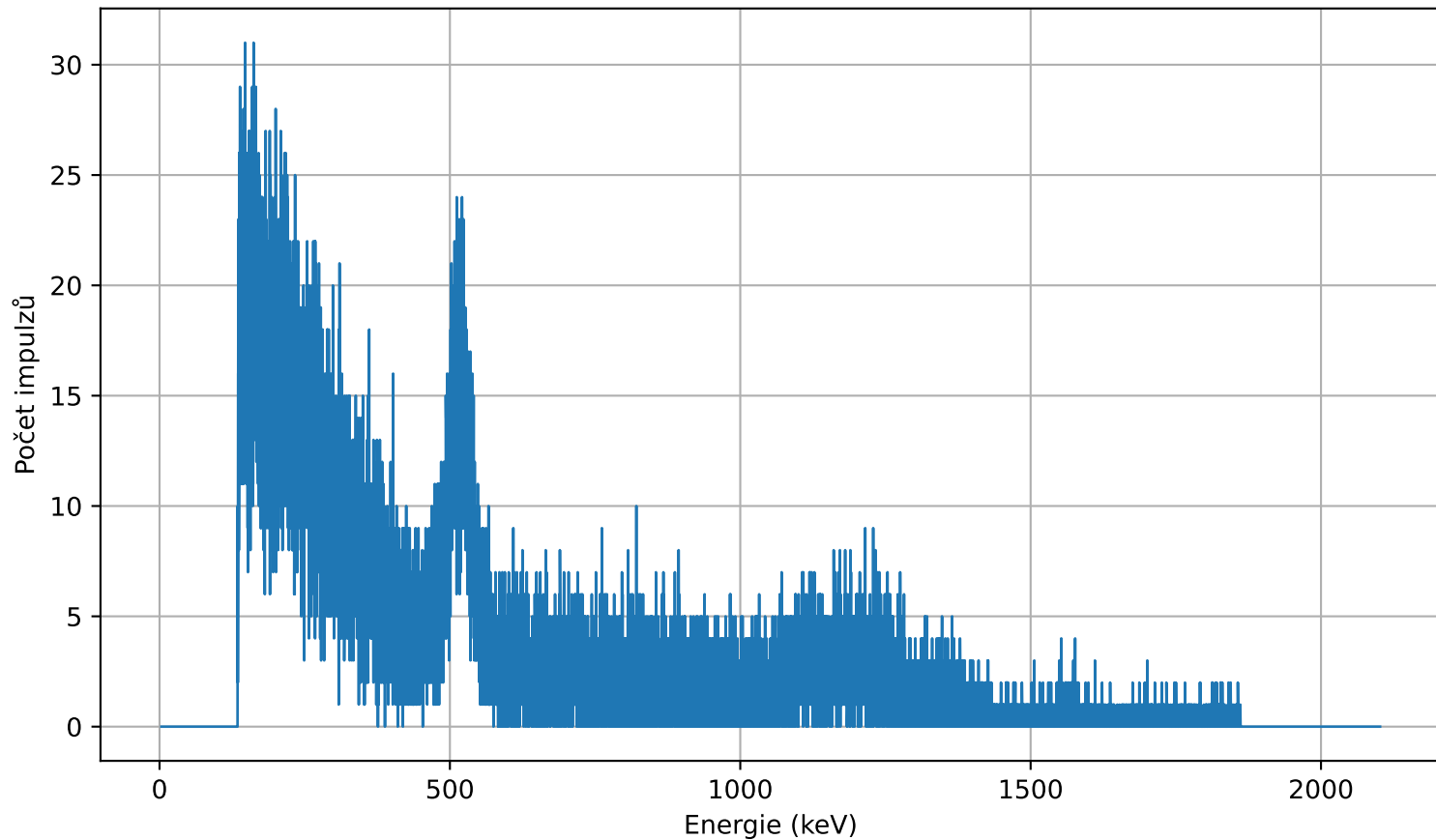
Gama spektrum (Sodík 22 - měření 1)
