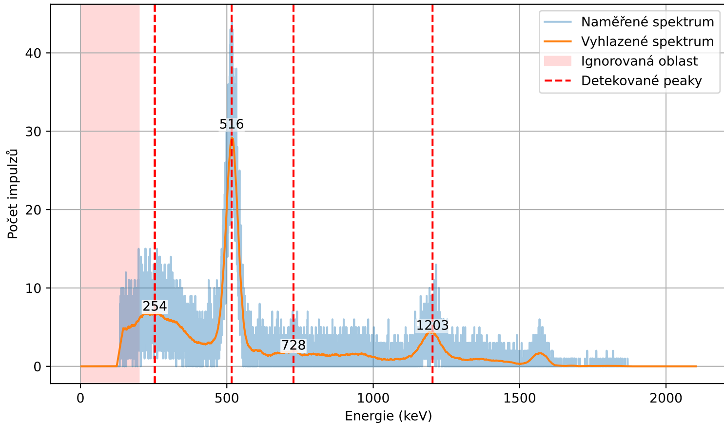
Gama spektrum (Sodík 22 - měření 2)
