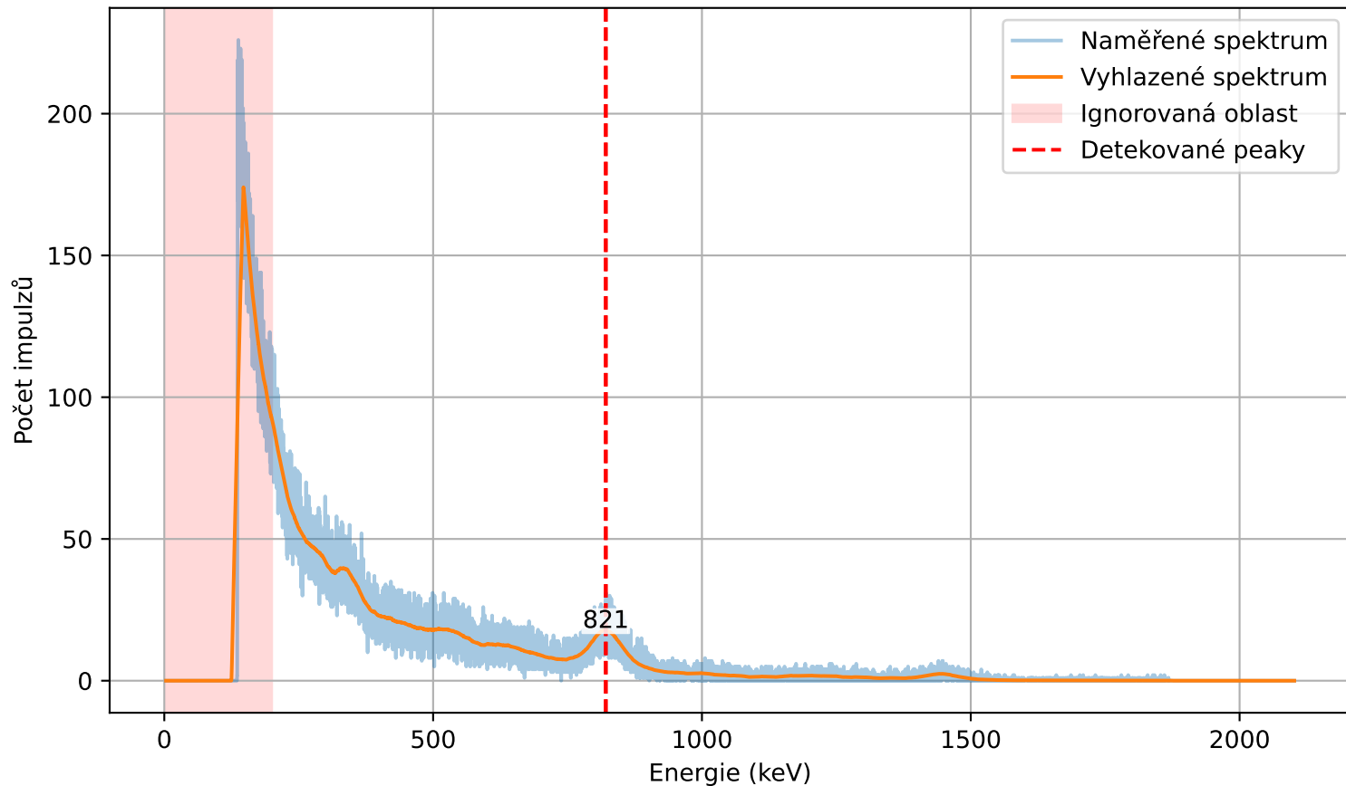
Gama spektrum (Pozadí)
