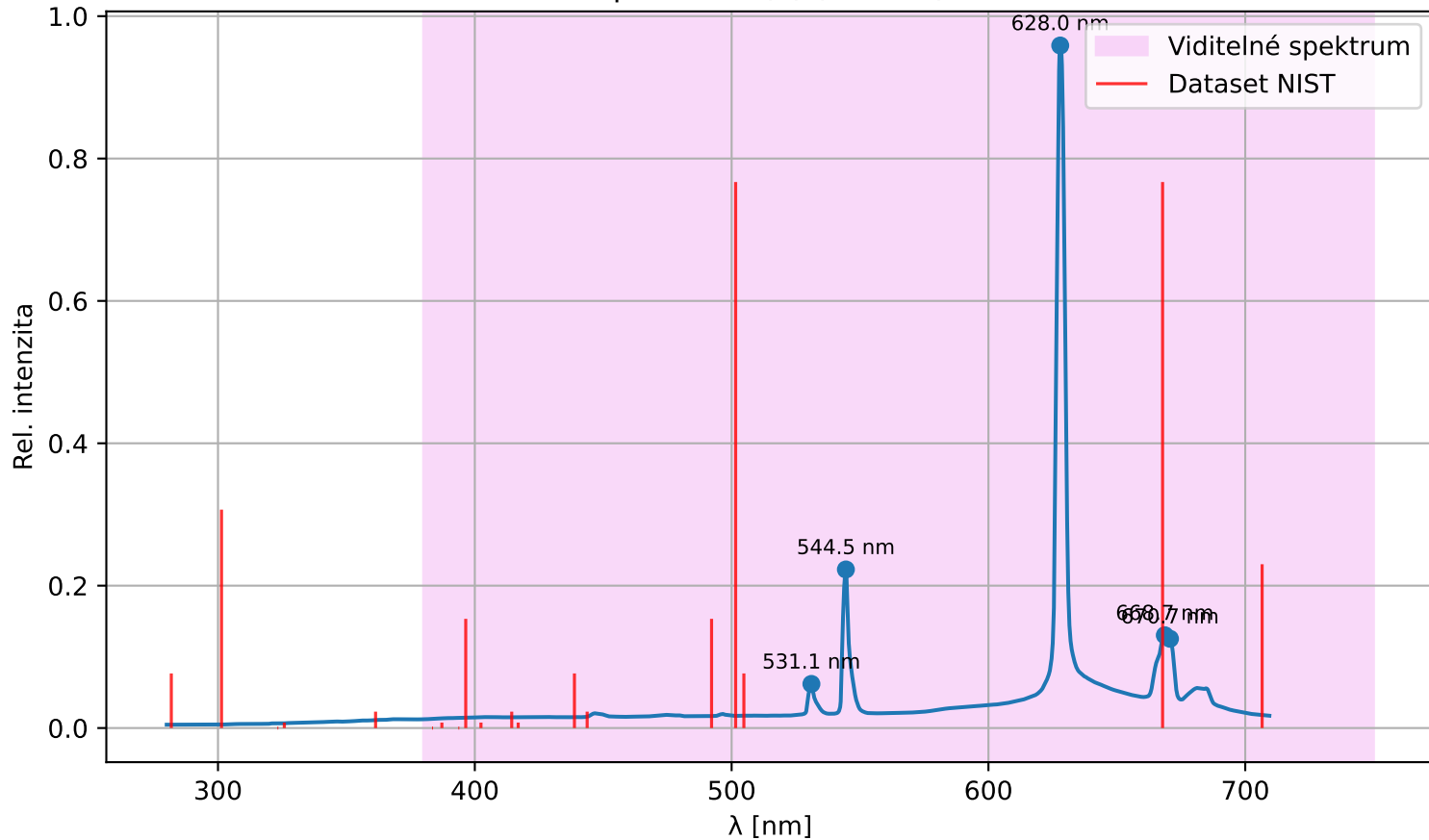
Spektrum I(\lambda) (Helium)
