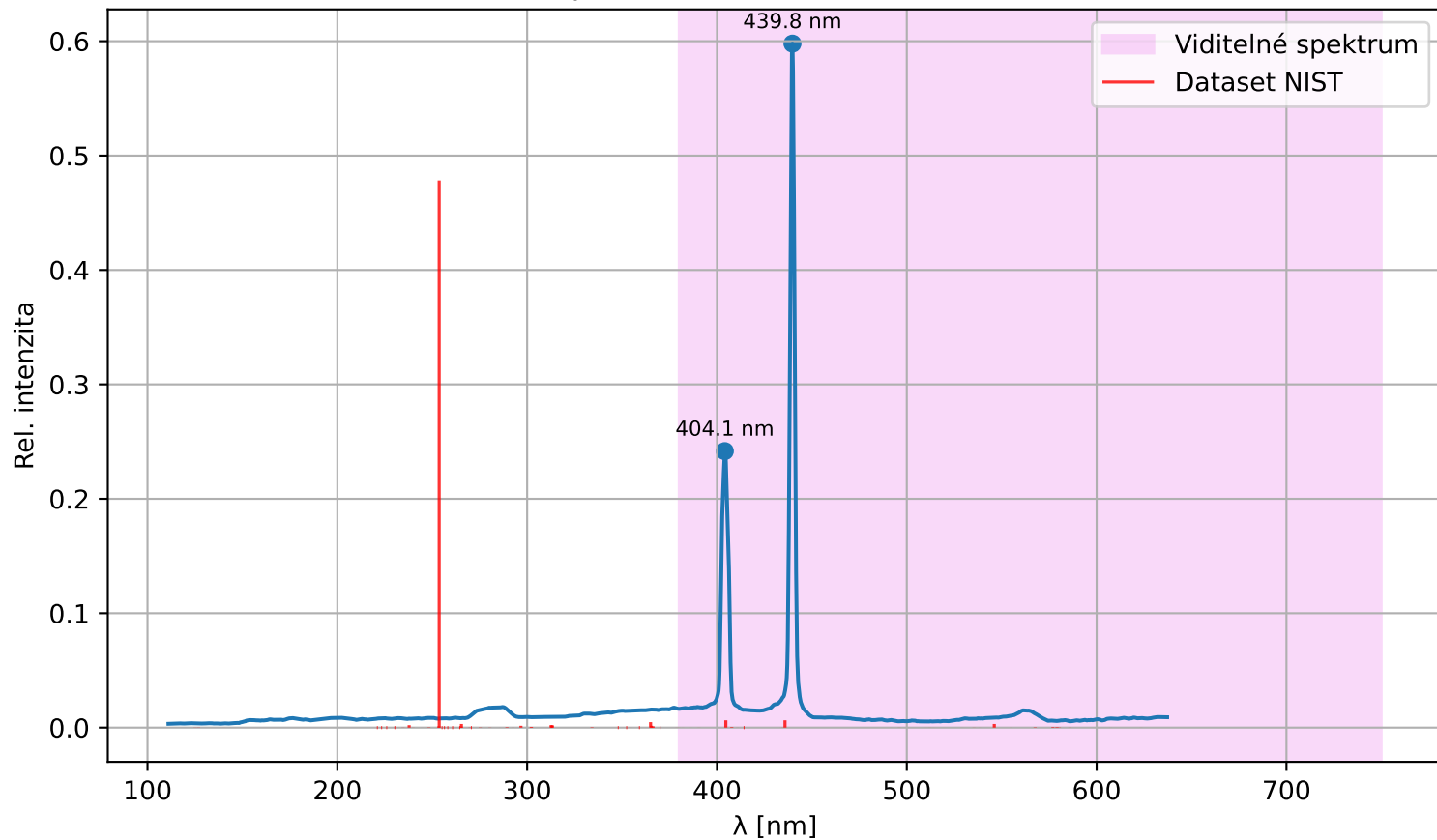
Spektrum I(\lambda) (Rtuť studená)
