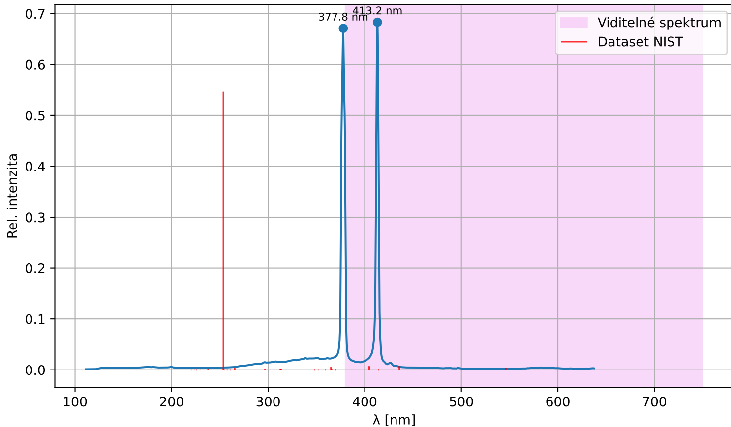
Spektrum I(\lambda) (Rtuť zahřátá)
