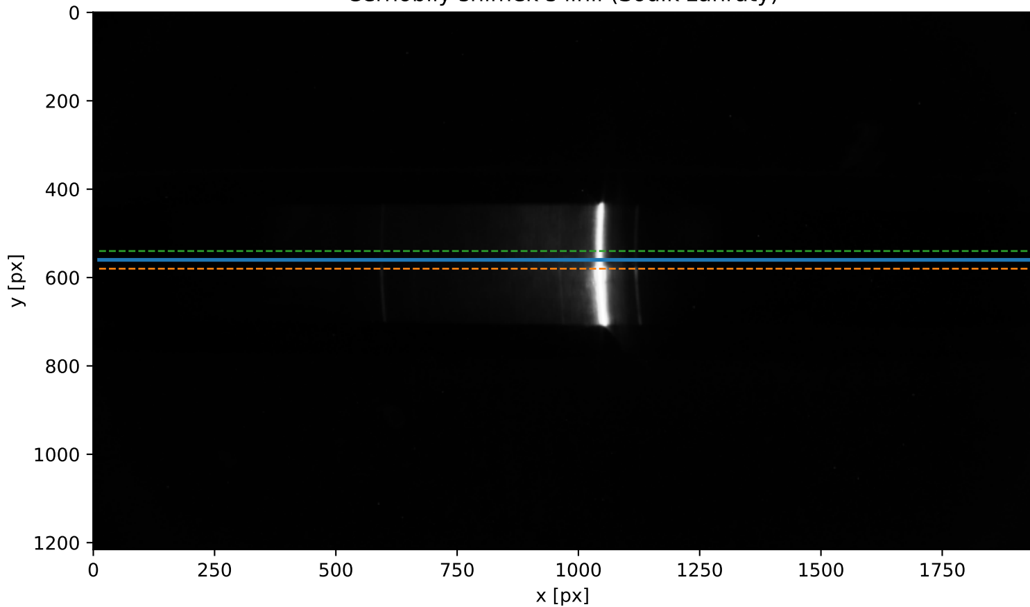
Černobílý snímek s linií (Sodík zahřátý)
