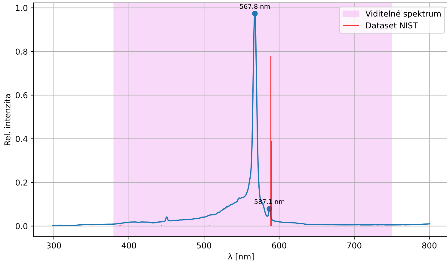
Spektrum I(\lambda) (Sodík zahřátý)
