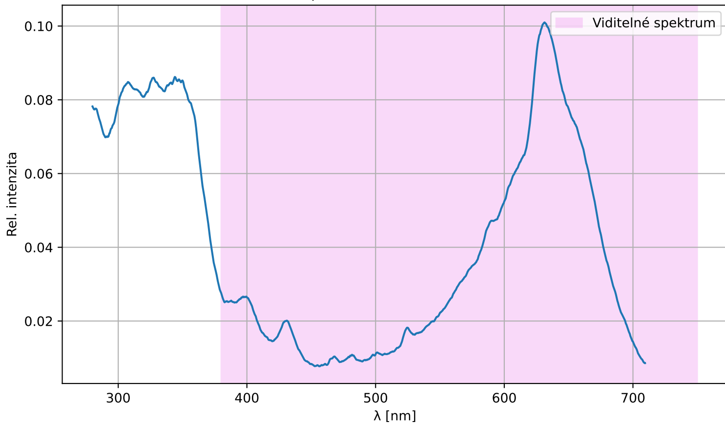
Spektrum I(\lambda) (Žárovka)
