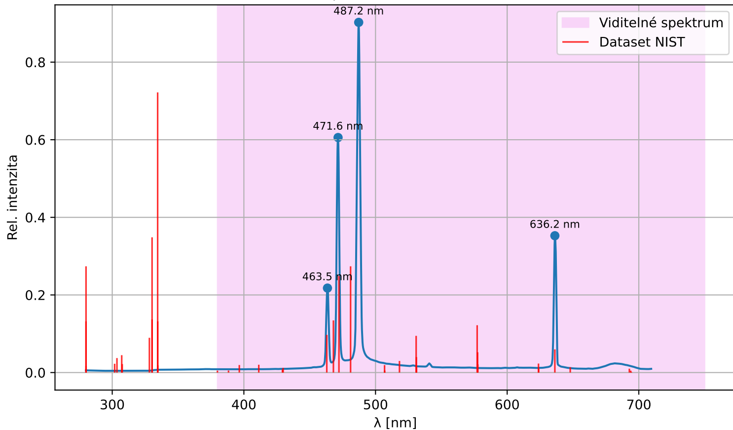
Spektrum I( \lambda ) (Zn)
