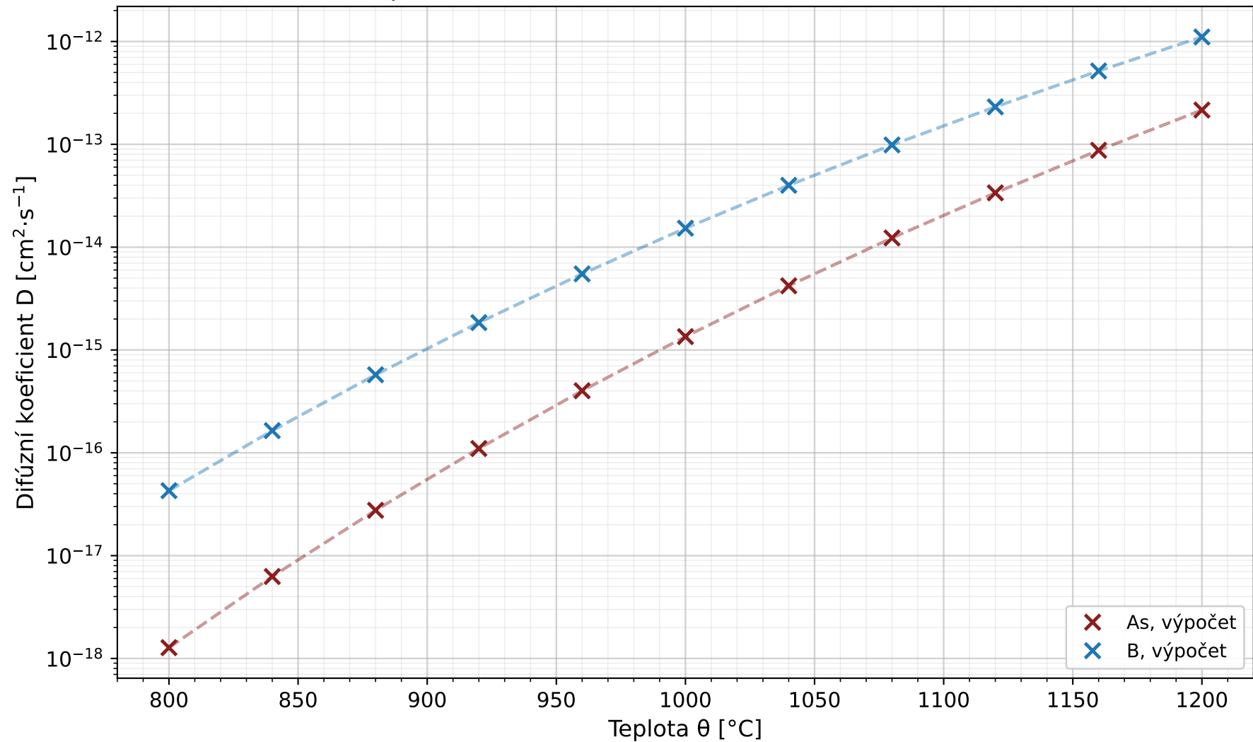
Teplotní závislost difúzního koeficientu v křemíku
