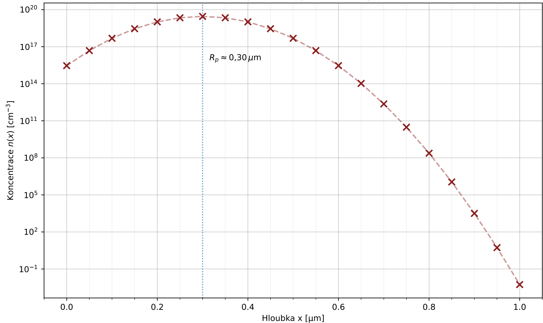
Koncentrační profil bóru po iontové implantaci
