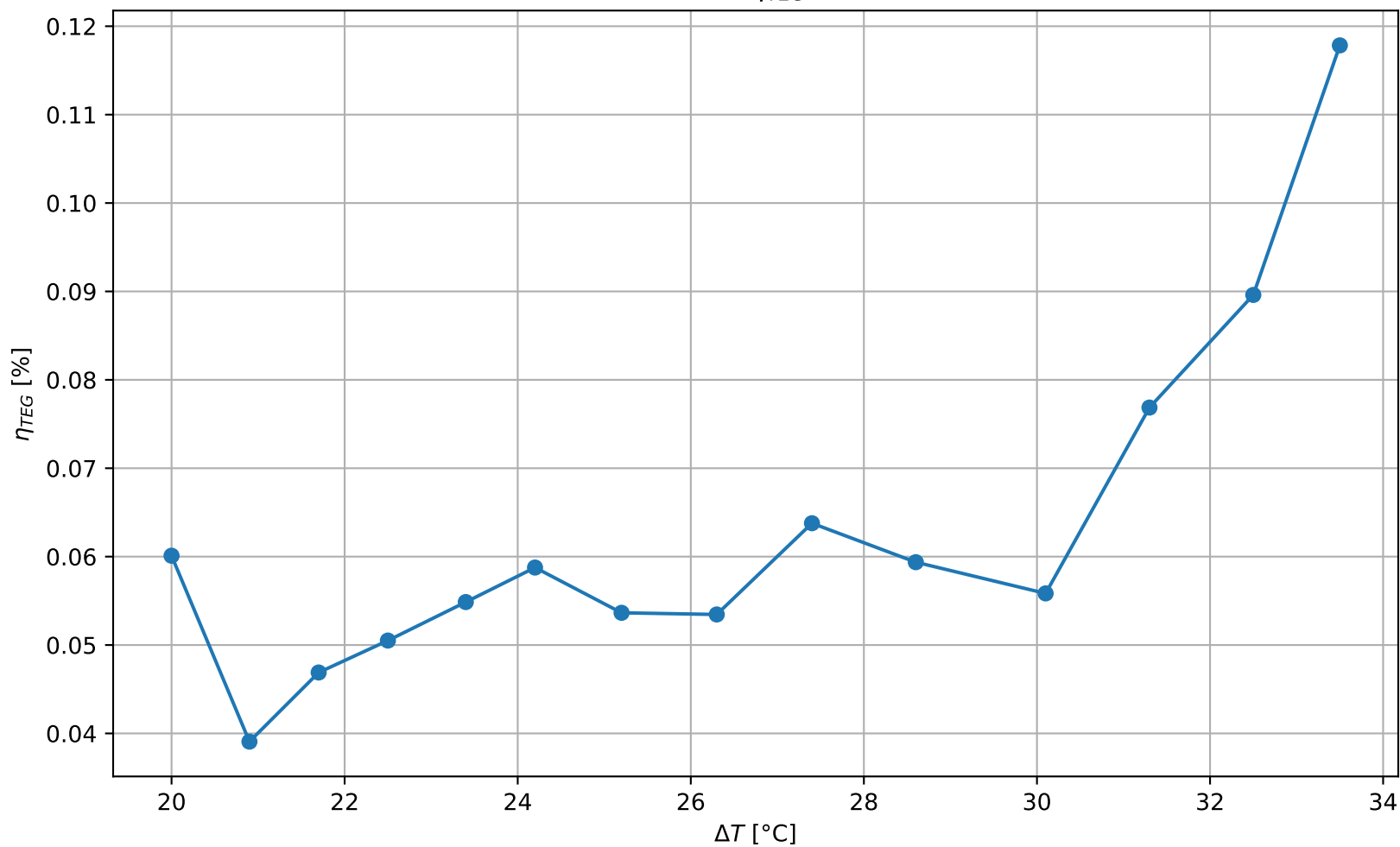
Závislost \eta_{TEG} na \Delta T
