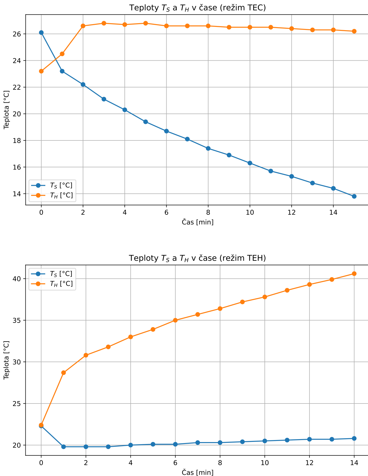
Obrázek 3: Grafy vývoje teplot na stranách termočlánku v čase
