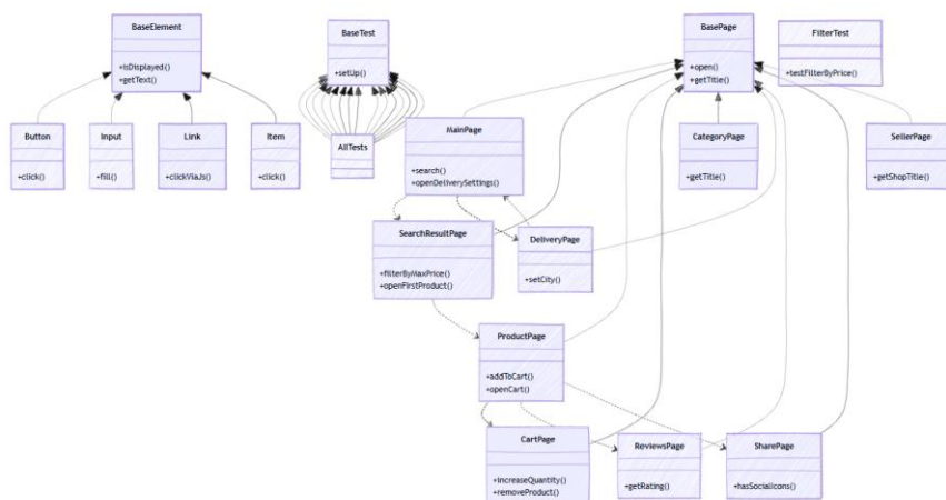
Рисунок 1 – UML-диаграмма классов тестового проекта
