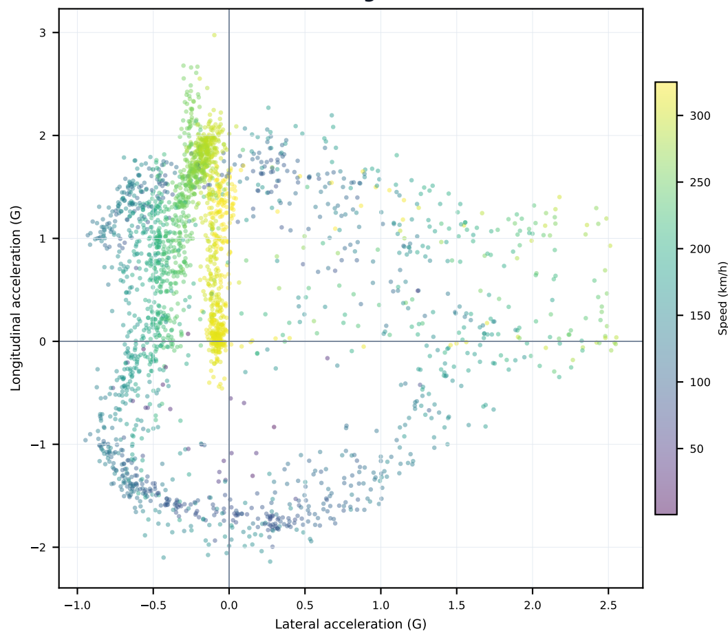
G-G Diagram
