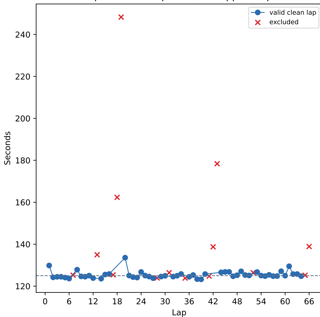
Lap-time development / Sviluppo tempi
