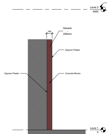
3 Section 2 1 : 20
