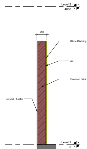
2 Section 1 1 : 20
