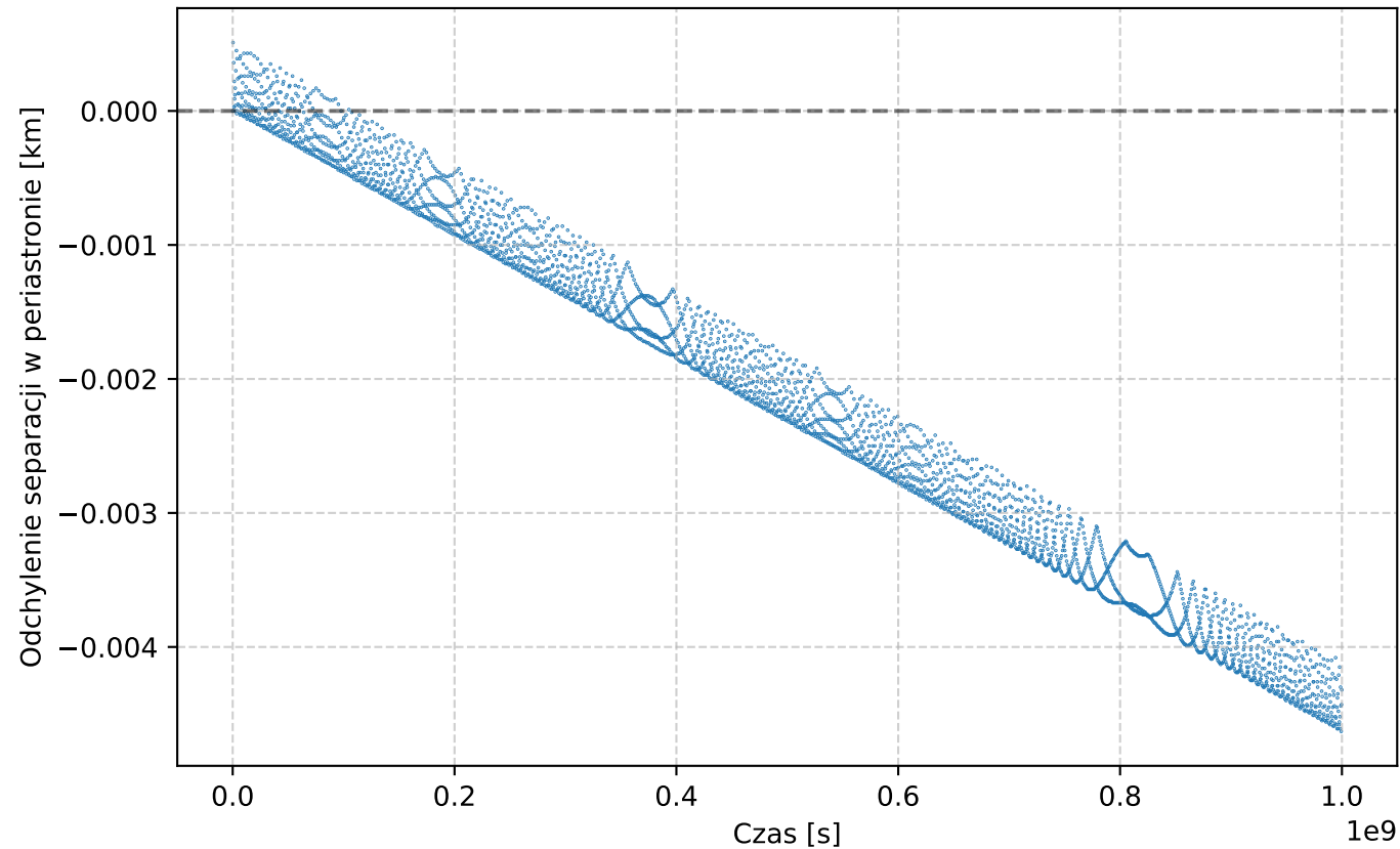
Zmiany separacji obiektów w periastronie względem początkowej wartości
