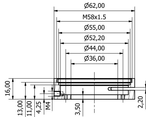
A-A ( 1 : 1 )
