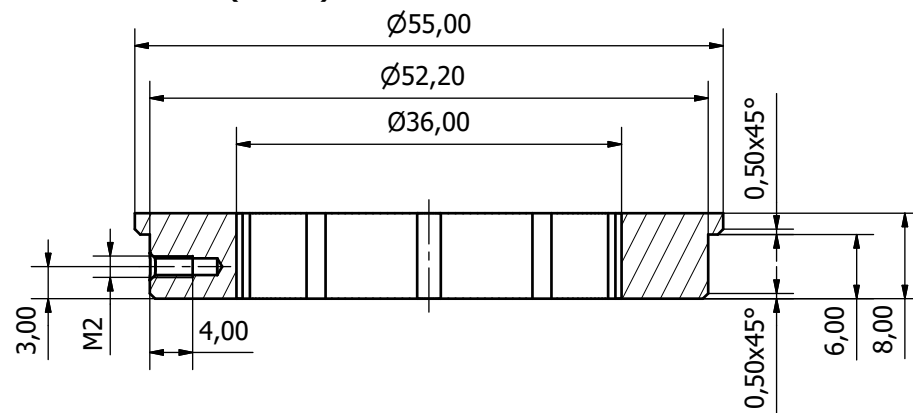
D-D ( 2:1 )
