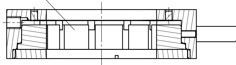
B - B ( 2 : 1 )
