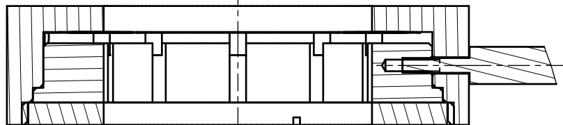
A - A ( 2 : 1 )
