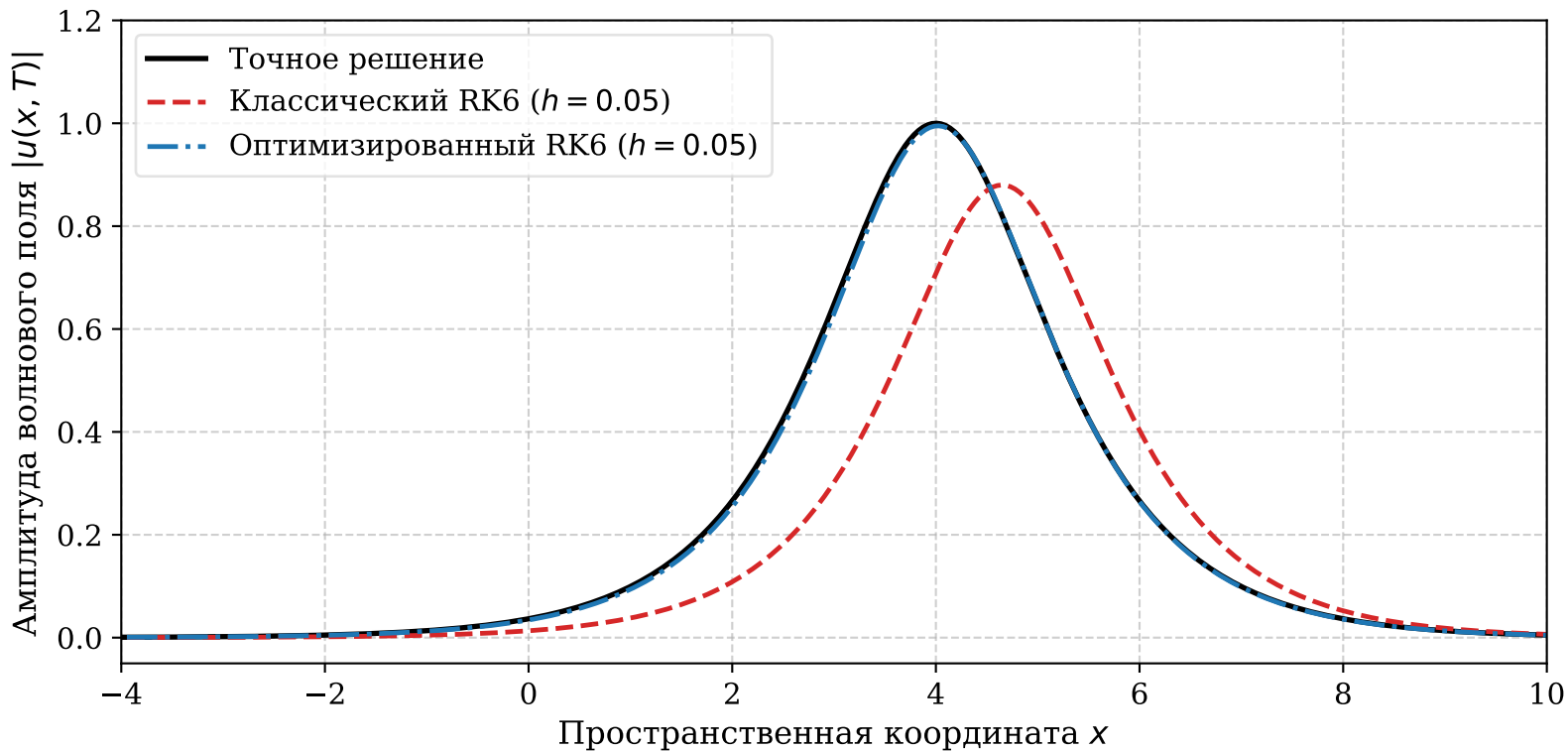
Сравнение профилей солитона в момент времени T = 2.0
