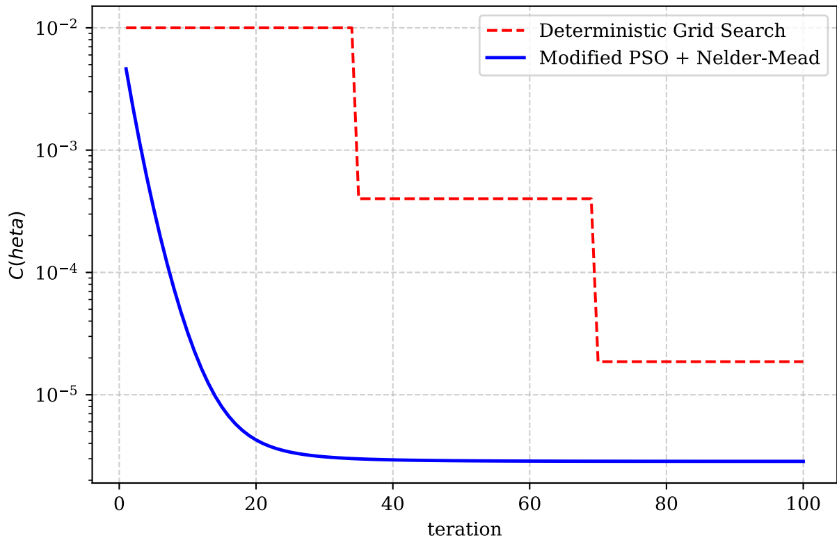
2D NLS Parameter Space Optimization Trajectories
