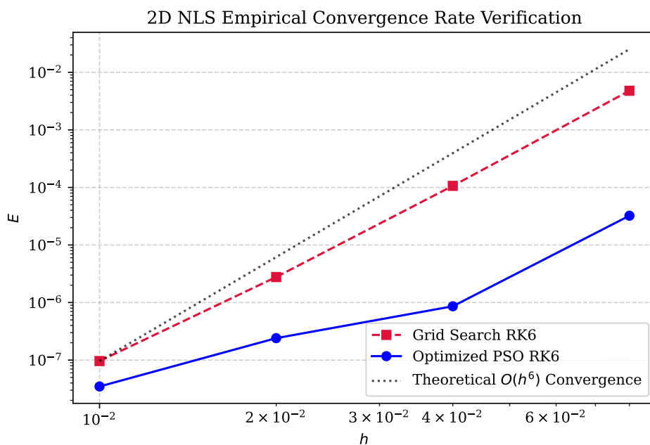
Рис. 6.3. Зависимость погрешности численной схемы от шага интегрирования
