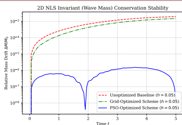
Консервативность схем
