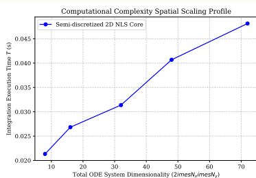
Пространственная масштабируемость
