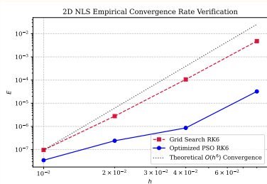
Порядок точности
