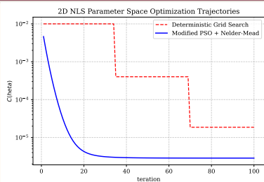
Сходимость алгоритмов
