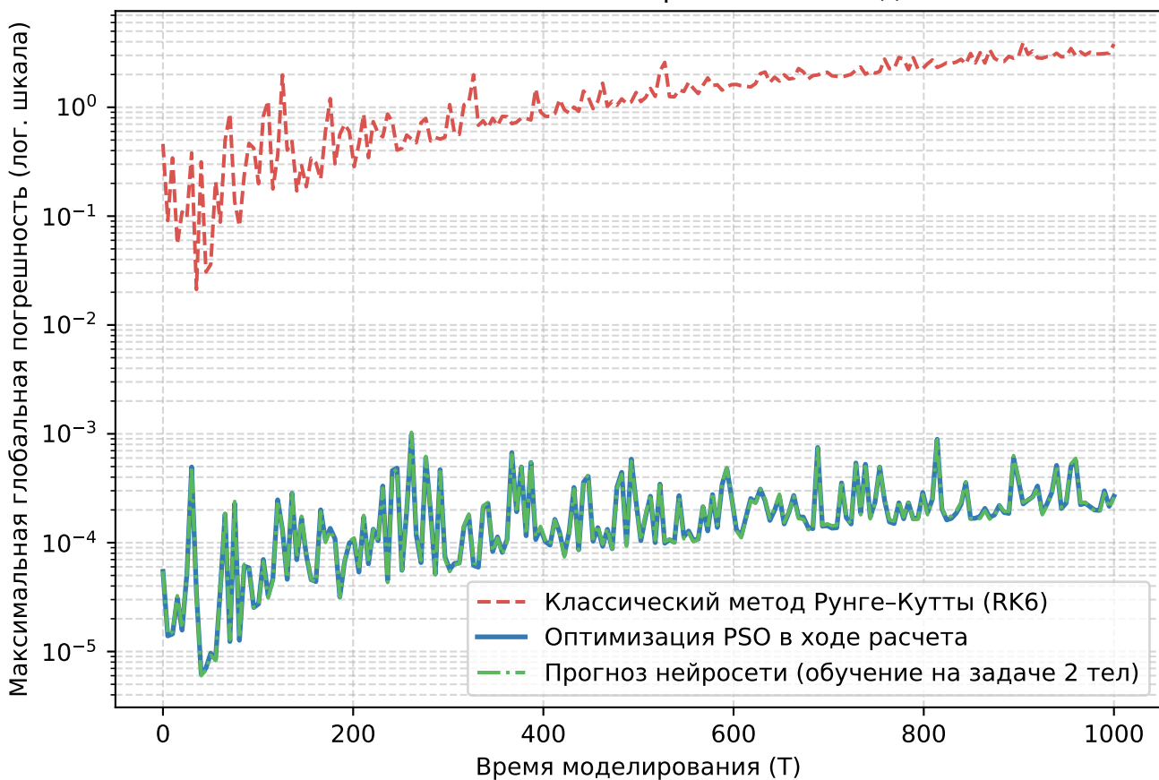
Накопление глобальной погрешности в задаче N тел
