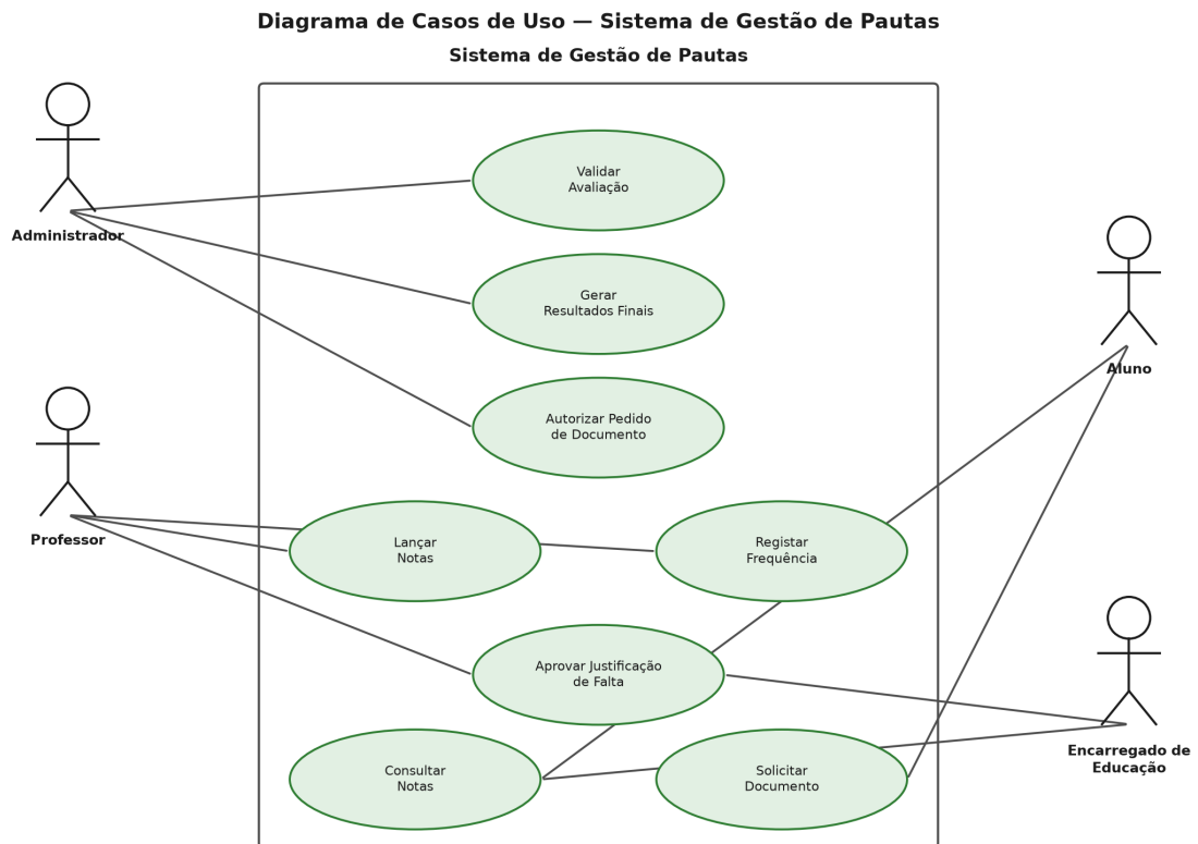
Figura 4 — Diagrama de Casos de Uso do Sistema de Gestão de Pautas
