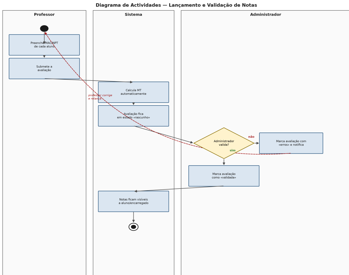
Figura 6 — Diagrama de Actividades: lançamento e validação de notas
