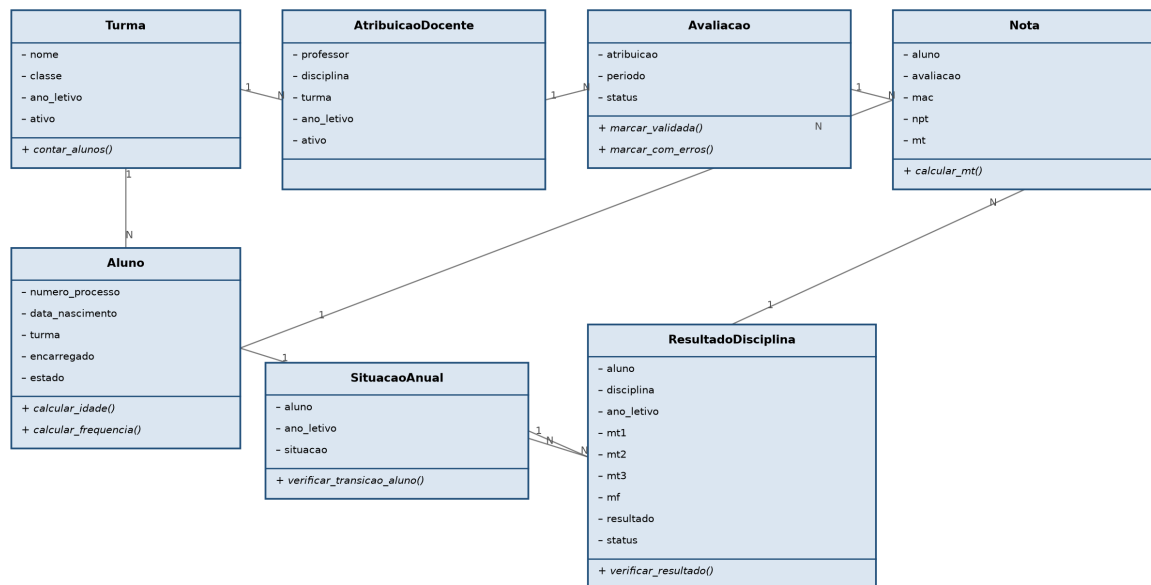
Diagrama de Classes (UML) — Domínio de Pautas
