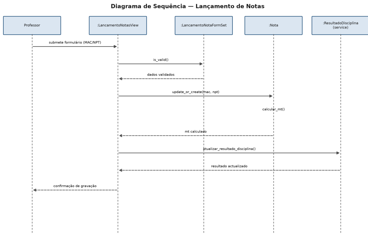
Figura 7 — Diagrama de Sequência: lançamento de notas
