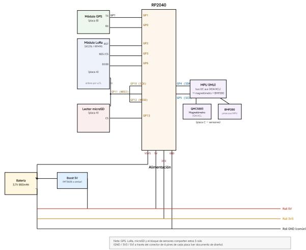
Esquemático – RP2040 + LoRa + GPS + SD + Sensores + Alimentación
