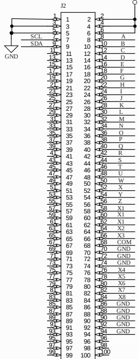
LSHM-150-06.0-L-DV-A-N-K-TR
