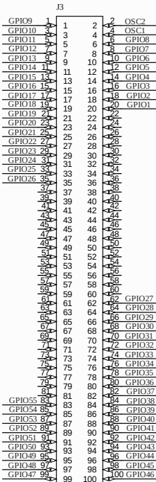
LSHM-150-06.0-L-DV-A-N-K-TR
