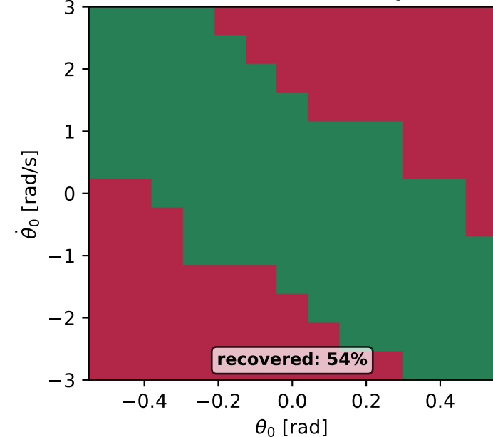
(d) cart-pole — value + L_{grad}
