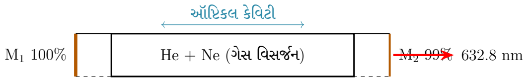
Figure 5.4: He-Ne લેસર: ઊંચી-પરાવર્તક કેવિટીમાં પ્રતિફલન-પ્રવર્ધન (Gain) દ્વારા સતત કિરણ.
