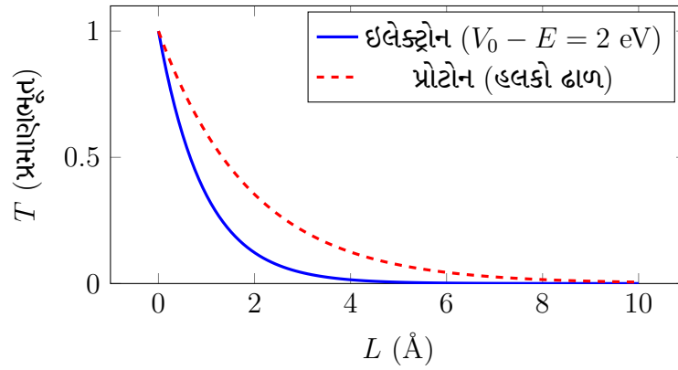
Figure 4.3: T \propto e^{-2\alpha L} — પહોળાઈ/ઢળ વધે તો ટનલિંગ પ્રચંડ રીતે ઘટે.
