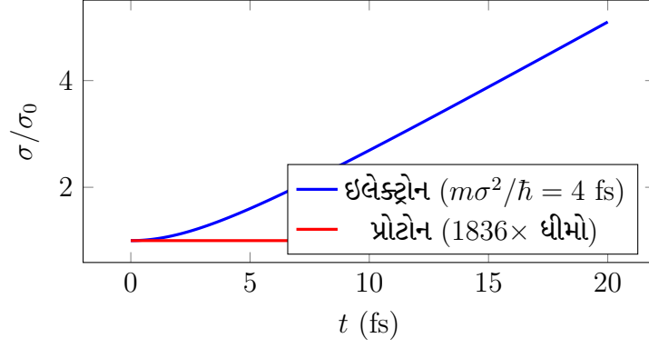
Figure 2.4: હલકા કણોનાં પેકેટ ઝડપથી ફેલાય છે; m \rightarrow \infty મર્યાદામાં શાસ્ત્રીય કણ મળે.
