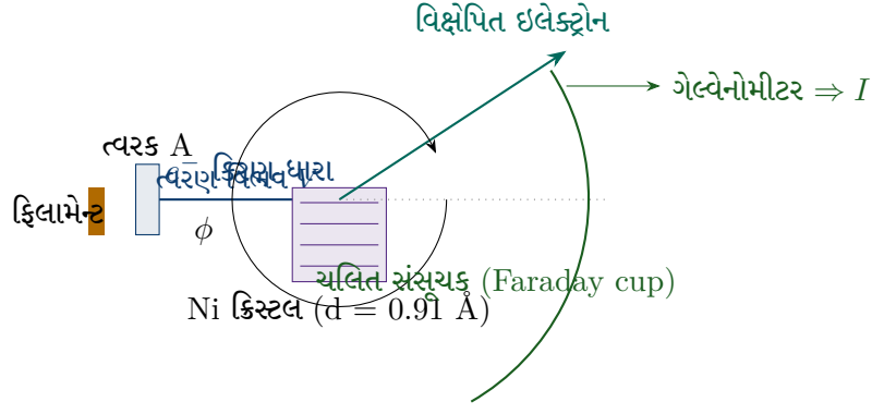
Figure 1.4: ડેવિસન-જર્મર પ્રયોગની યોજના: ત્વરિત ઇલેક્ટ્રોન Ni ક્રિસ્ટલ પર વિદ્યુત કણો થાય છે; સંસૂચક કોણ \phi બદલાવી તીવ્રતા માપે છે.
