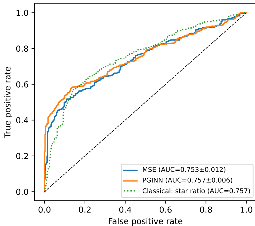
1 locus, n=10
