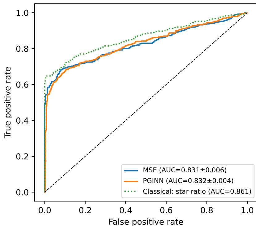
1 locus, n=10
