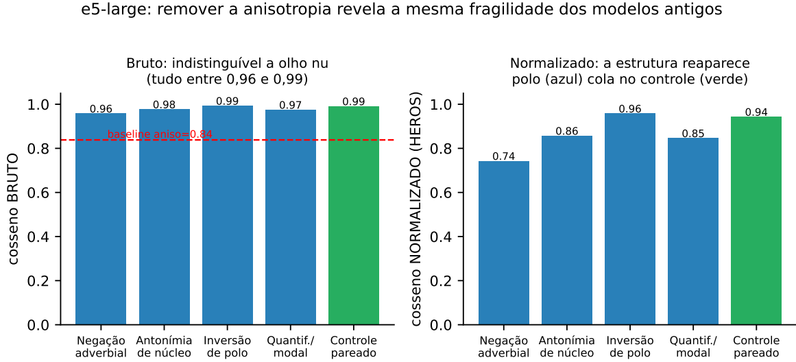
Figura 2: O achado central. À esquerda, o que o operador vê: cosseno bruto do e5, uniforme perto de 0,99. À direita, o que de fato ocorre: removida a anisotropia, a inversão de polo (azul) praticamente não se separa do controle de paráfrase (verde). A fragilidade estava lá, oculta pela geometria.
