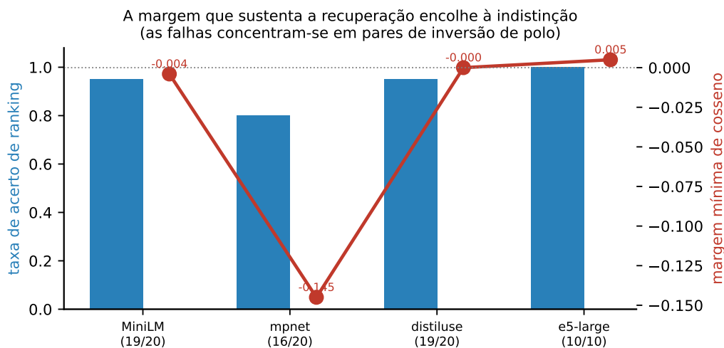
Figura 3: Recuperação por modelo. O acerto de ranking é alto em todos, mas a margem mínima de cosseno que sustenta esses acertos (em vermelho) estreita-se até o limiar da indistinção; no e5, cujo cosseno absoluto vive todo perto de 0,99, a margem mínima é de cinco milésimos. As falhas dos modelos abertos concentram-se, ademais, em pares de inversão de polo.
