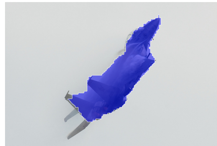
PicoSAM2
