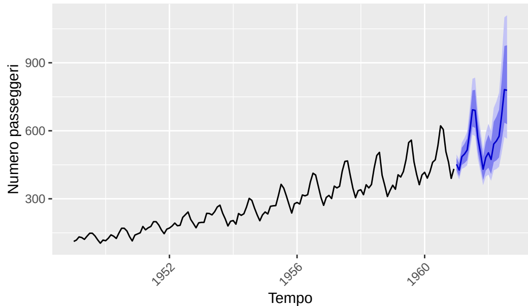
Predizione ARIMA(0,1,1)(0,1,1)[12]
