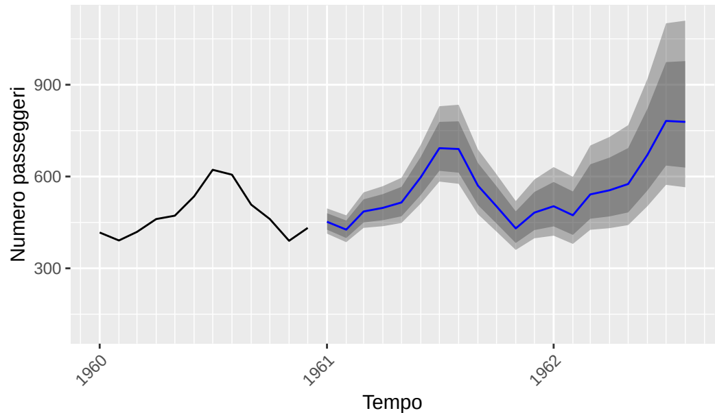
Predizione ARIMA(0,1,1)(0,1,1)[12]
