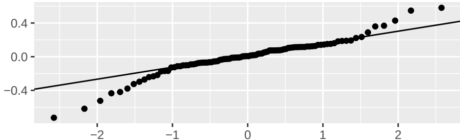
Grafico Q-Q
