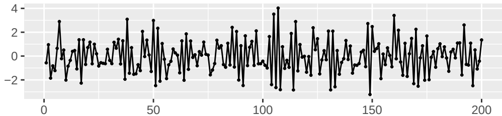
Serie MA
