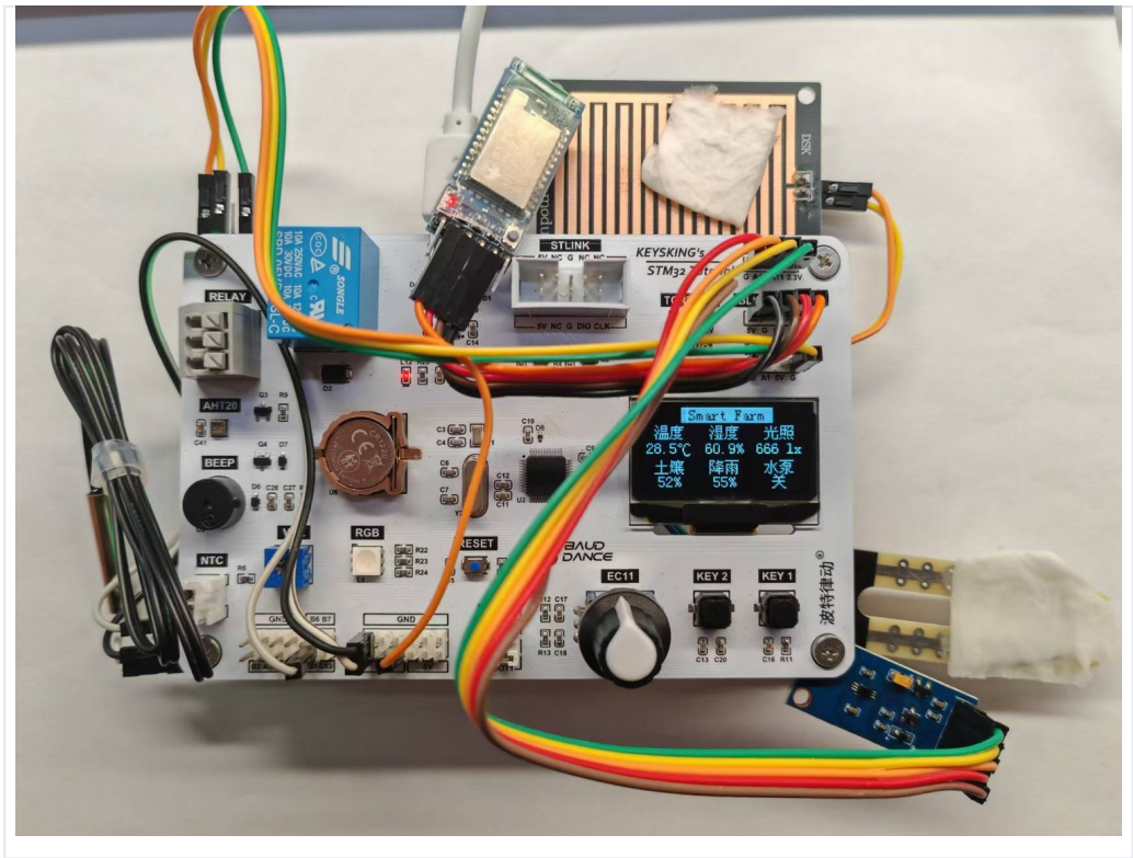
图 2-2 OLED 实时显示温湿度、光照与土壤湿度等多路传感数据
