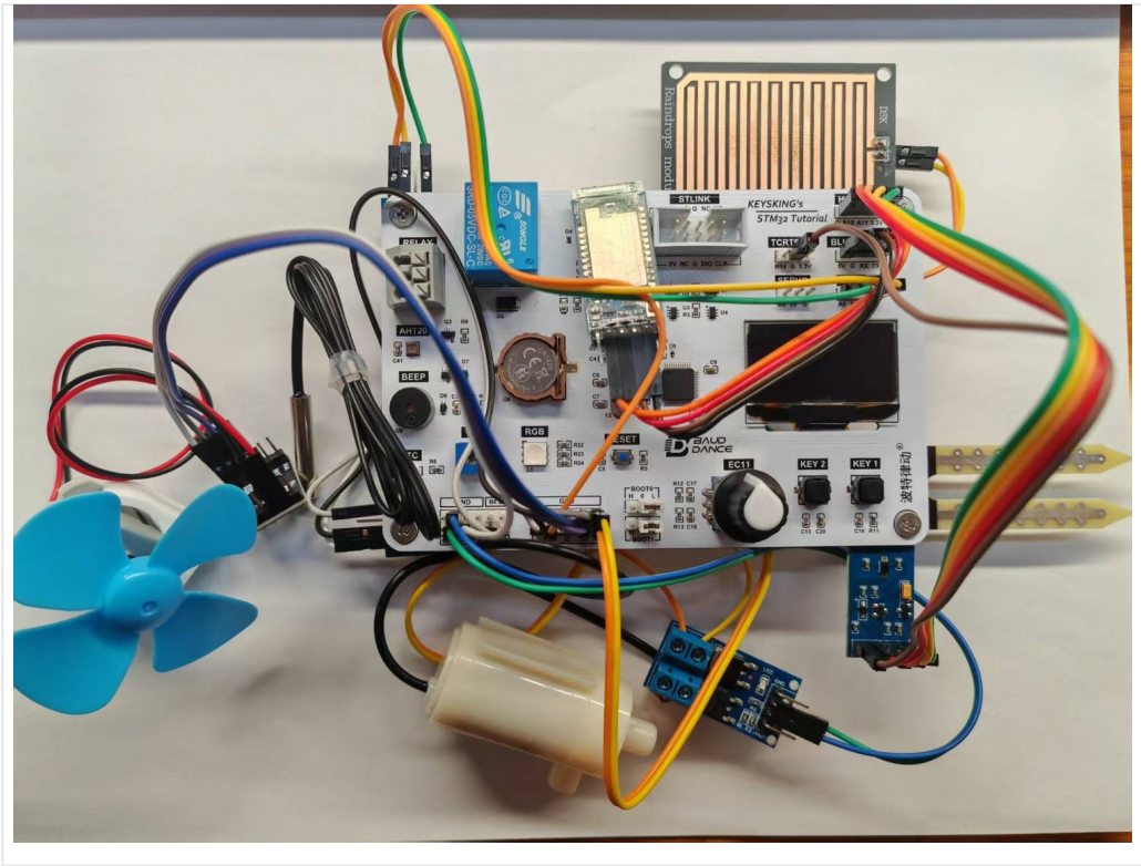
图 2-1 智慧农场系统整机：多源传感器、OLED、水泵与 PWM 风扇执行器
