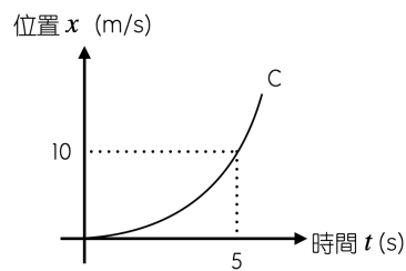
C：等加速度運動
