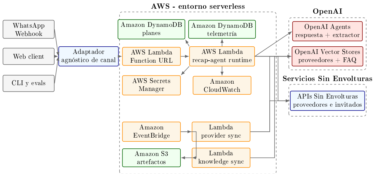
Figura 1: Vista de despliegue AWS y relación con canales, OpenAI y APIs de Sin Envolturas. Colores: gris para canales, naranja para cómputo AWS, verde para datos, rojo para OpenAI y azul para APIs externas.
