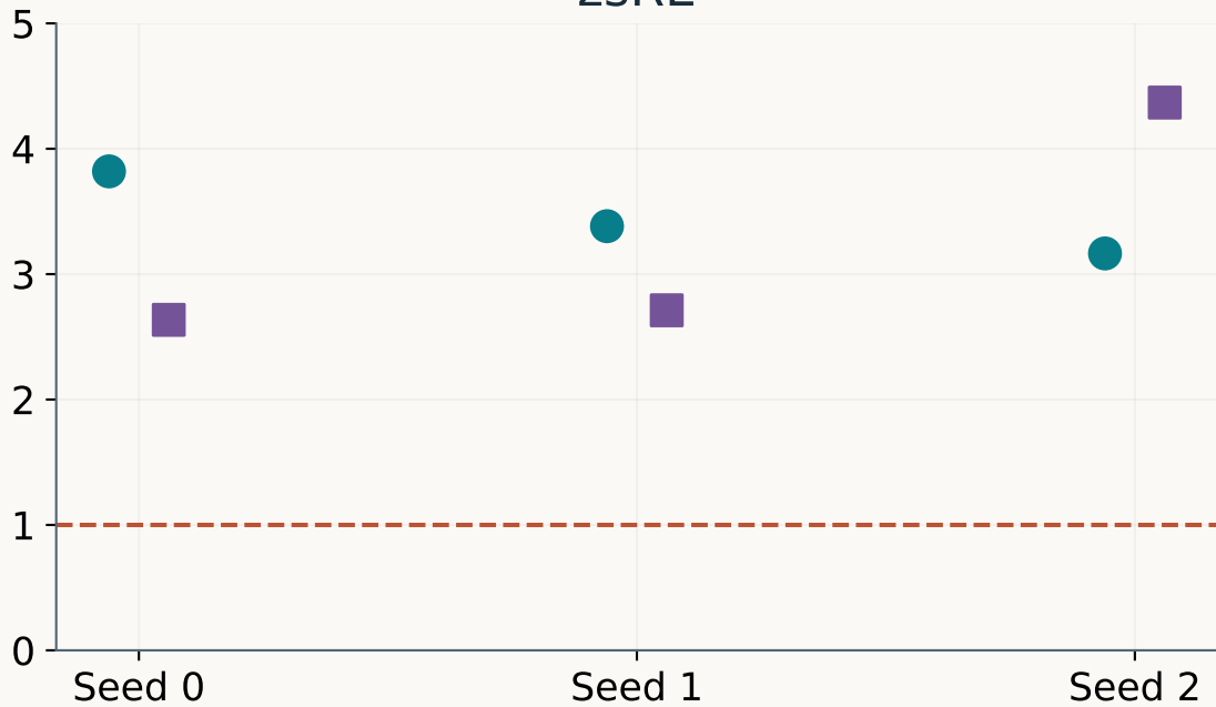
zsRE
