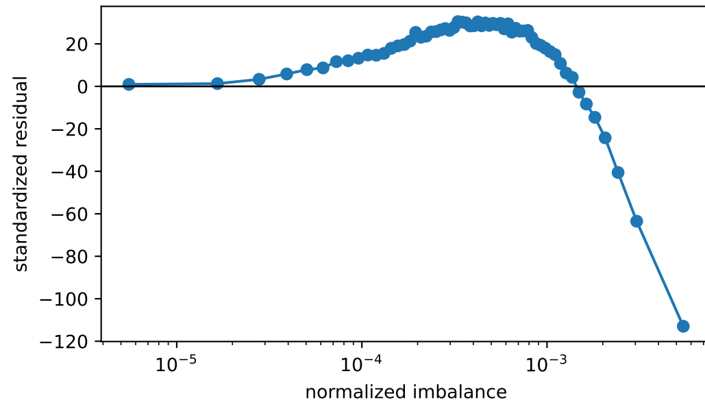
linear
