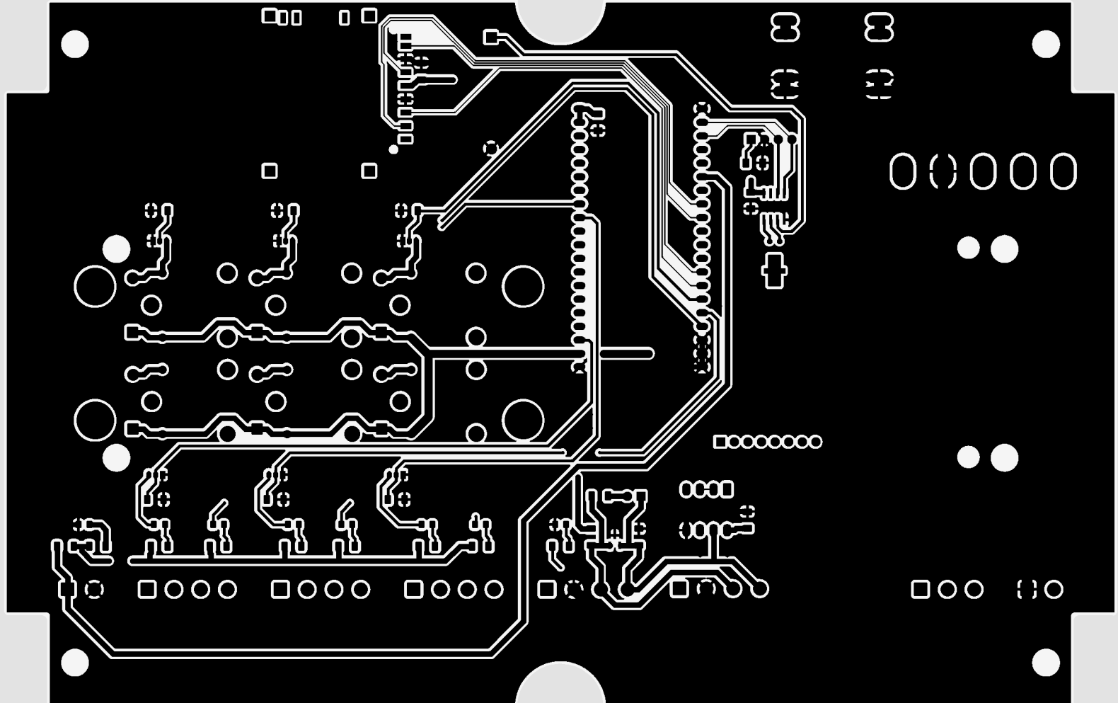
E1784060 TOP layer Image (topview)
