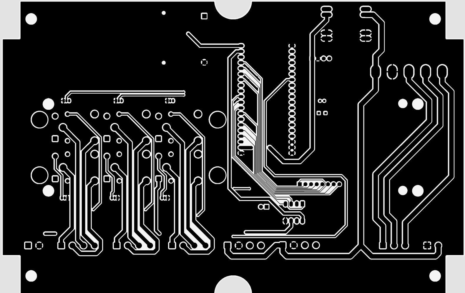
E1784060 BOTTOM layer Image (topview)
